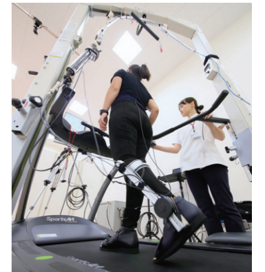
人工筋肉駆動式足関節ロボット
